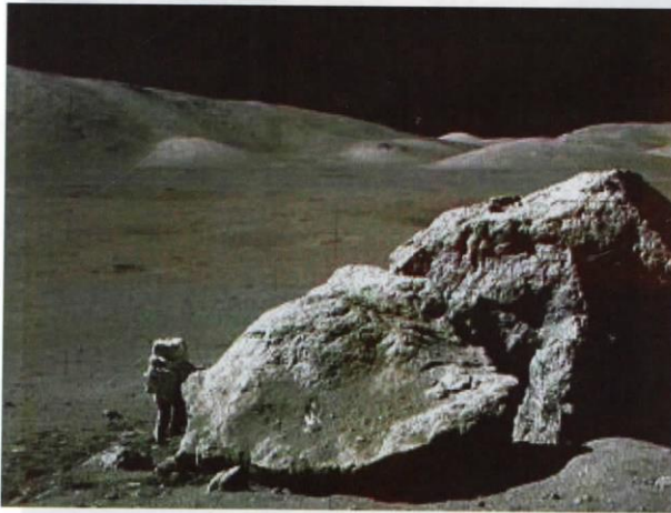
[رائد الفضاء والجيولوجي (هاريسون سميث) إيَّان بعثة (أبوللو ١٧) عام ١٩٧٢. انظر [ سطح القمر ]
