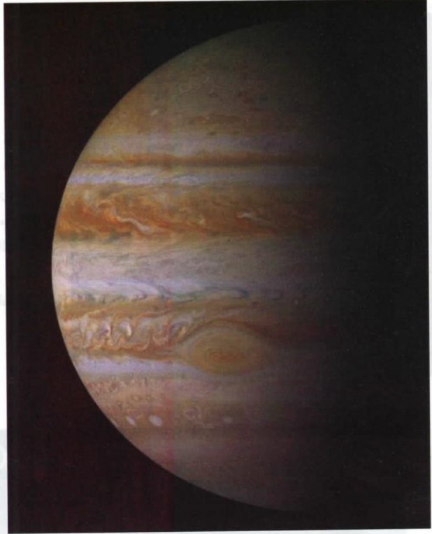
صورة مركبة من مجموعة من الصور الملتقطة إبان تحليق المركبة (كاسينى) فوق المُشْتَرَى عام ٢٠٠٠. انظر [المُشْتَرَى]
