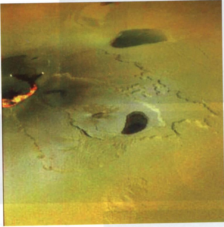
اندلاع بركانيّ على سطح القمر (إيو) على نحو ما رصده عام ٢٠٠٠ المركبة (جاليليو). انظر [توابع المُشترى]
