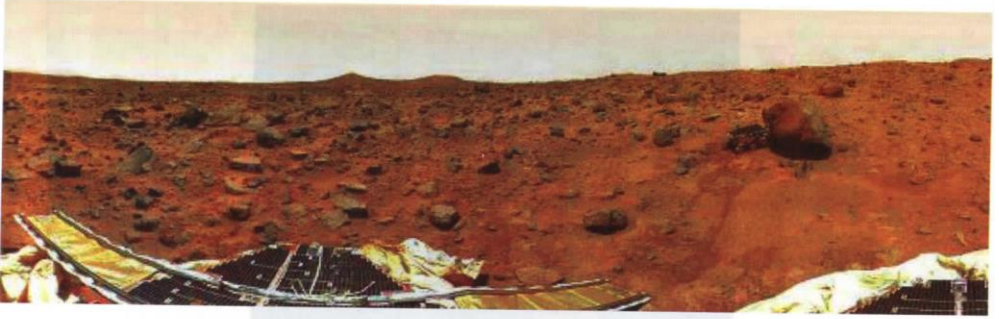
بانوراما لسطح المريخ منقطة إبان بعثة (بانثايندر) عام ١٩٩٧. انظر [ كوكب المريخ ]
