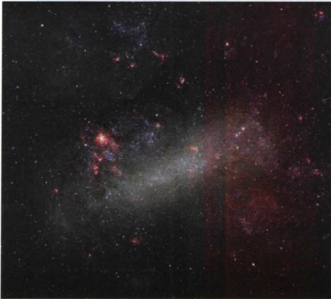
السحابة الماجلَانِيَّة الكبرى وهى المَجْرَة غير المنتظمة التابعة لمجرتنا درب التبانة والموجودة على بعد مائة وستين ألف سنة ضوئية من الأرض، والتي يصل قطرها إلى نحو ثلاثين ألف سنة ضوئية. انظر [مختلف أنواع المجرات]
