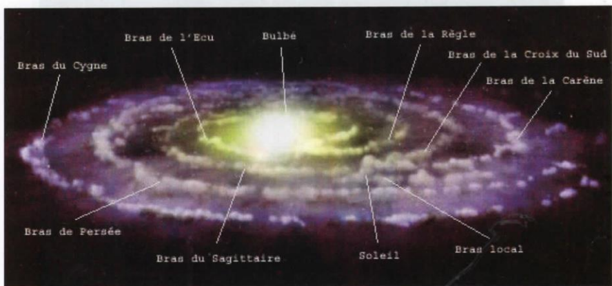
رؤية تخيلية للمجرة مستوحاة من عمليات رصد في نطاق الأشعة تحت الحمراء وموجات الراديو. انظر [المجرة]
