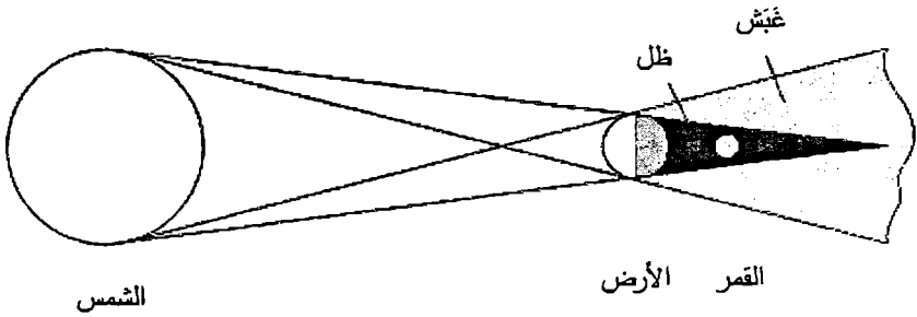
خسوف للقمر يحدث إبان مرور الأرض بين الشمس والقمر.
