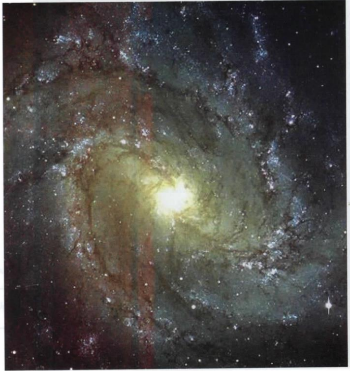
المجرة الحلزونية القضيبيّة (ميسييه ٣٣) الموجودة على بُعد خمسة عشر مليون سنة ضوئية فى كوكبة الحوّية. انظر [الأذرع الحلزونية]
