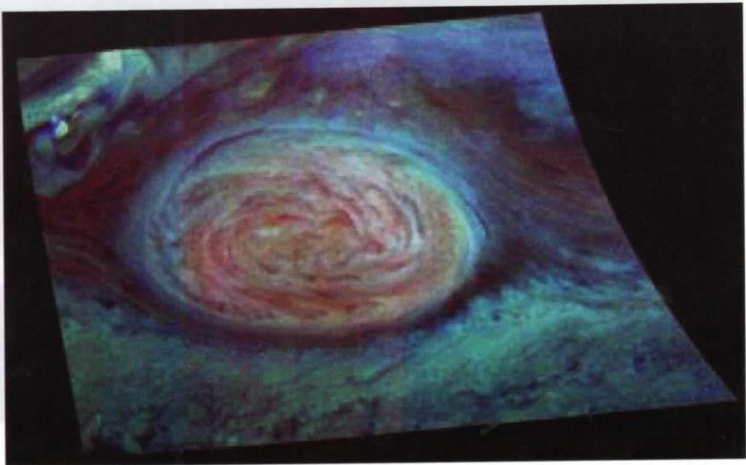
صورة بألوان غير حقيقية للبقعة الحمراء الكبرى فى كوكب المُشْتَرَى التقطتها المركبة (جاليليو) فى مجال الأشعة تحت الحمراء عام ١٩٩٦. انظر [المُشْتَرَى]
