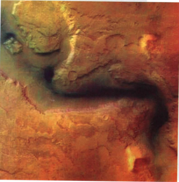
صورة لحوض (هيلا) على كوكب المريخ منقطة بأداة التصوير HRSC بالمرحلة الأوروبية (مَارِس إكسبريس). ويمكننا تبيّن قناة اسمها (رويال فاليس)، وهي على الأرجح نتاج تدفقات مائية منذ مليارات السنين. انظر [ المياه على المريخ ]
