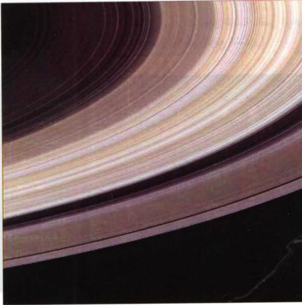
صورة لحلقات زُحل التقطتها المركبة (كاسيني) قبل تسعة أيام من دخولها في مدار على مسافة (٦,٤) مليون كيلومتر. وتتكون الحلقات بالأساس من ثلوج المياه. وترجع اختلافات الألوان على الأرجح إلى اختلاف درجات تداخل عناصر أخرى مثل الصخور ، على سبيل المثال. انظر [الكوكب زُحل]
