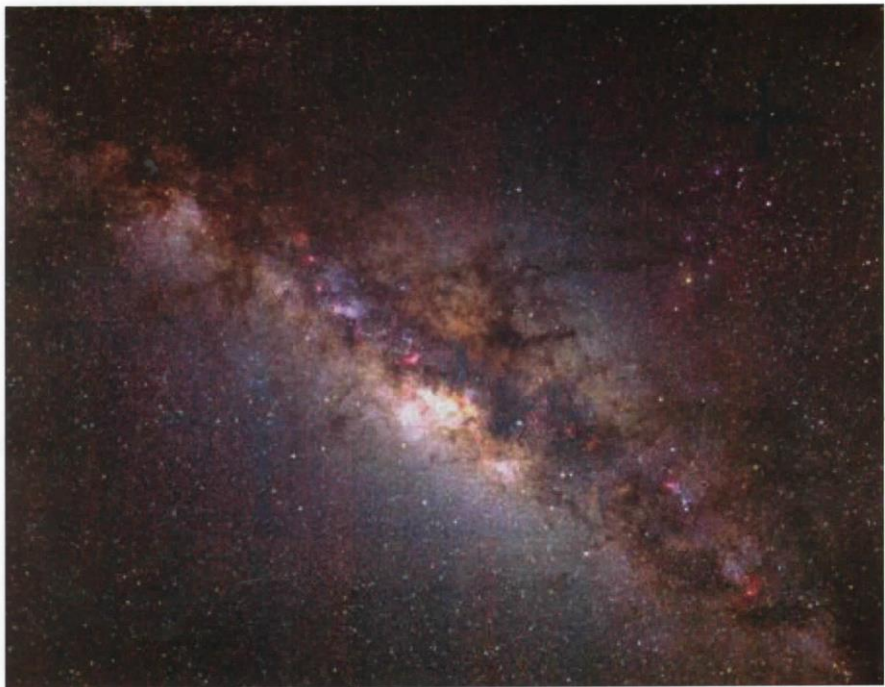
مشهد خلّاب لمجرّتنا درب التبانة في الصيف. انظر [دراسة تاريخية لدرب التبانة]
