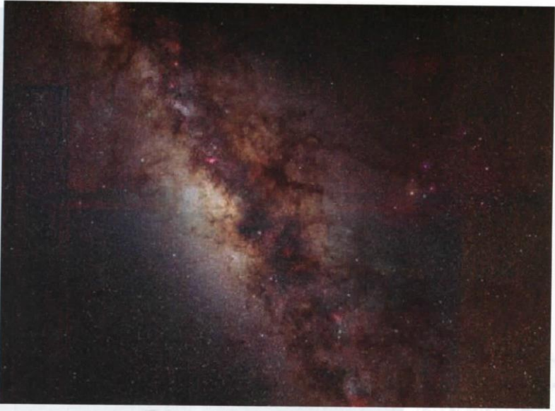
مشهد في اتجاه مركز درب التبانة في كوكبة القوس. انظر [المركز المجري]
