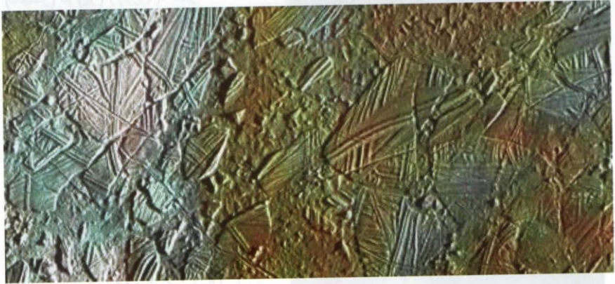
السطح المُكوّن من التلوج المُهشّمة للقمر (أوروبا) التابع لكوكب المُشترى. وترجع اختلافات الألوان إلى ترسّبات الجسيمات الدقيقة من التلوج. والصورة مركبة من مجموعة من الصور التّقطت خلال عمليات رصد قامت بها المركبة (جاليليو) بين عاميّ ١٩٩٦ و ١٩٩٧. انظر [أقمار المُشترى]
