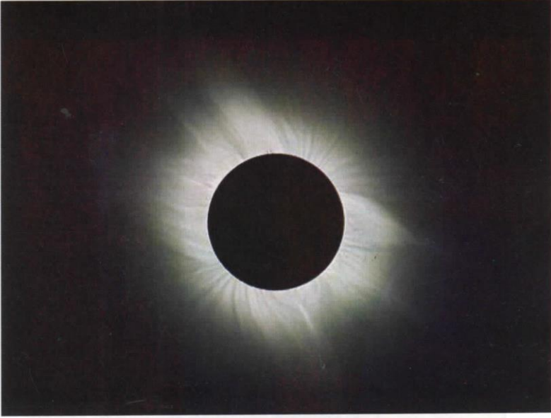
(الكورونا) أو الهالة الشمسية التي ظهرت إبان كسوفٍ للشمس في مارس عام ٢٠٠٦ في تركيا. انظر [الكروموسفير والهالة والرياح الشمسية]
